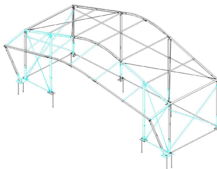
9m conversion kit highlighted
